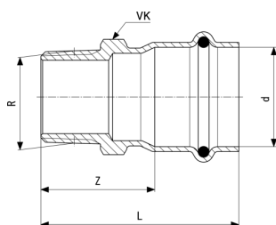
Prestabo-přechodový kus - nelegovaná ocel, pozinkováno model 1111
