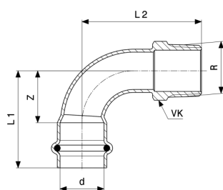
Prestabo-přechodový oblouk 90° - nelegovaná ocel, pozinkováno model 1114
