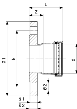
Prestabo-přírubový přechod - nelegovaná ocel, pozinkováno model 1159.1
