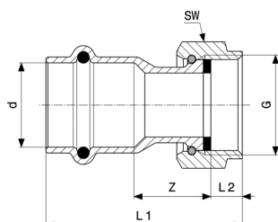
Prestabo-připojovací šroubení - nelegovaná ocel, pozinkováno model 1163
