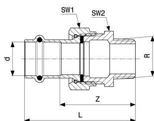
Prestabo-přechodové šroubení - nelegovaná ocel, pozinkováno model 1165
