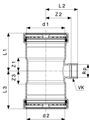
Prestabo XL-T-kus - nelegovaná ocel, pozinkováno model 1117.2XL
