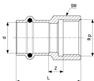
Prestabo-přechodový kus - nelegovaná ocel, pozinkováno model 1112
