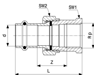
Prestabo-přechodové šroubení - nelegovaná ocel, pozinkováno model 1162
