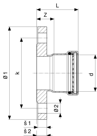
Prestabo XL-přírubový přechod - nelegovaná ocel, pozinkováno model 1159XL
