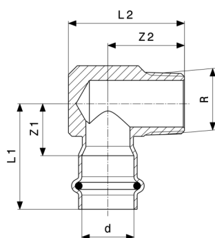
Prestabo-přechodové koleno 90° - nelegovaná ocel, pozinkováno model 1114.1
