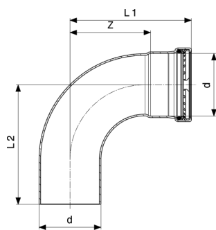
Prestabo XL-oblouk 90° - nelegovaná ocel, pozinkováno model 1116.1XL
