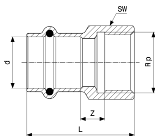
Prestabo-přechodový kus - nelegovaná ocel, pozinkováno model 1112
