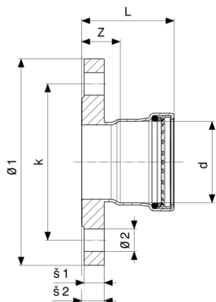
Prestabo XL-přírubový přechod - nelegovaná ocel, pozinkováno model 1159.1XL
