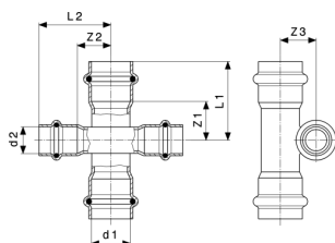
Prestabo-křížová tvarovka - nelegovaná ocel, pozinkováno model 1148
