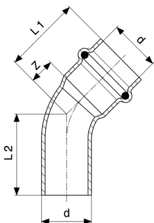
Prestabo-oblouk 45° - nelegovaná ocel, pozinkováno model 1126.1
