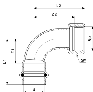
Prestabo-přechodový oblouk 90° - nelegovaná ocel, pozinkováno model 1114.5
