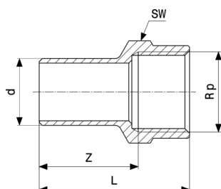
Prestabo-zásuvný kus - nelegovaná ocel, pozinkováno model 1112.1
