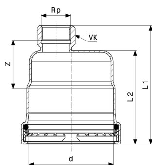
Prestabo XL-víčko - nelegovaná ocel, pozinkováno model 1156XL
