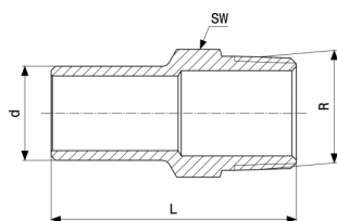
Prestabo-zásuvný kus - nelegovaná ocel, pozinkováno model 1111.1
