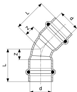
Prestabo-oblouk 45° - nelegovaná ocel, pozinkováno model 1126
