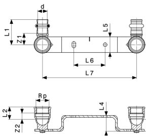
Sanpress-Montageeinheit Modell 2222
