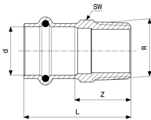
Sanpress-Übergangsstück - Rotguss oder Siliziumbronze Modell 2211
