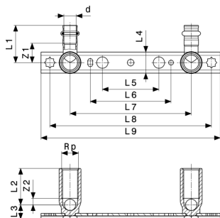
Sanpress-Montageeinheit Modell 2221
