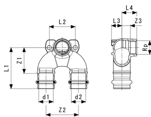
Sanpress-Doppelwandscheibe - Rotguss oder Siliziumbronze Modell 2228.7
