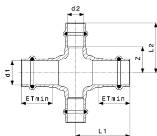
Sanpress-Kreuzungsstück - Rotguss oder Siliziumbronze Modell 2244
