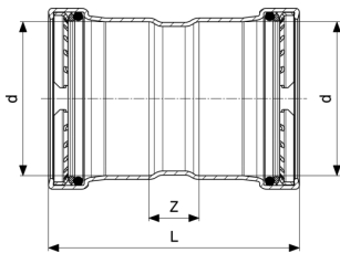
Profipress XL-Muffe - Kupfer Modell 2415XL
