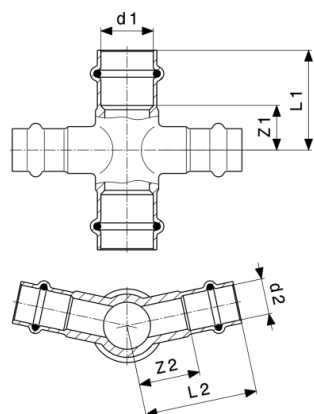
Sanpress-Kreuzstück 24° - Rotguss Modell 2247
