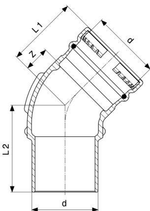
Sanpress XL-Bogen 45° - Rotguss Modell 2226.1XL
