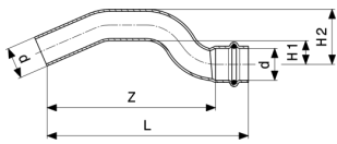
Profipress-Überbogen - Kupfer Modell 2427
