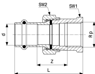
Sanpress-Übergangverschraubung - Rotguss oder Siliziumbronze Modell 2262
