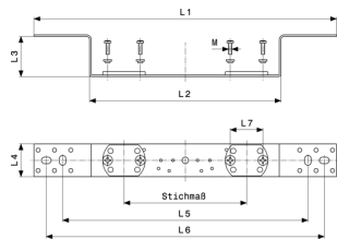
Halterung - Stahl verzinkt Modell 2021.7
