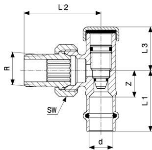
Sanpress-Rücklaufverschraubung - Rotguss Modell 2272.1
