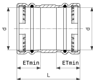
Sanpress XL-Schiebemuffe - Rotguss Modell 2215.5XL
