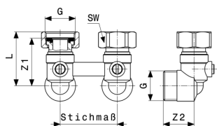
Heizkörperanschlussstück - Messing matt-vernickelt Modell 1097.5
