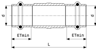
Sanpress-Schiebemuffe - Rotguss oder Siliziumbronze Modell 2215.5
