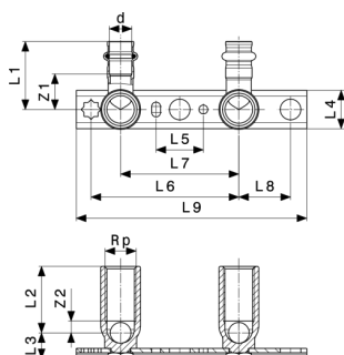
Sanpress-Montageeinheit Modell 2221.1
