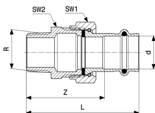
Sanpress-Übergangverschraubung - Rotguss oder Siliziumbronze Modell 2265
