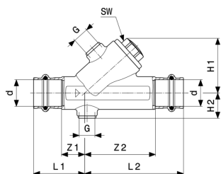
Easytop-Rückflussverhinderer Modell 2239.4
