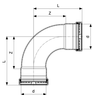
Profipress XL-Bogen 90° - Kupfer Modell 2416XL
