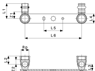
Sanpress-Montageeinheit Modell 2222.05
