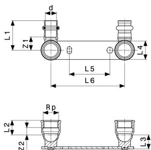
Sanpress-Montageeinheit Modell 2222.2
