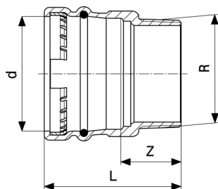
Sanpress XL-Übergangsstück - Rotguss Modell 2211XL
