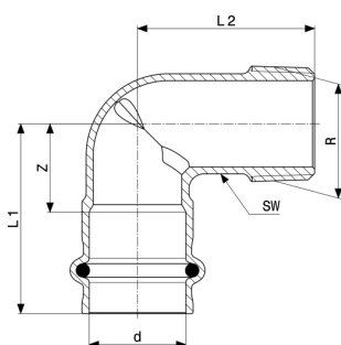
Sanpress-Übergangsbogen 90° - Rotguss oder Siliziumbronze Modell 2214
