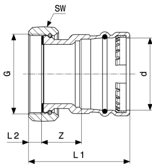
Sanpress XL-Anschlussverschraubung - Rotguss Modell 2263XL
