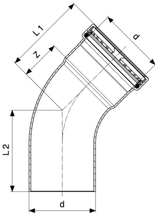
Profipress XL-Bogen 45° - Kupfer Modell 2426.1XL
