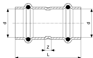
Profipress-Muffe - Kupfer Modell 2415
