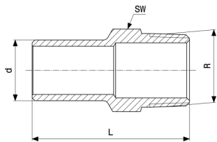
Sanpress-Einsteckstück - Rotguss oder Siliziumbronze Modell 2211.1
