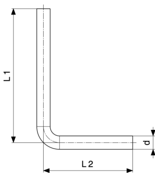
Anschlussbogen 90° - Edelstahl Modell 2271.1
