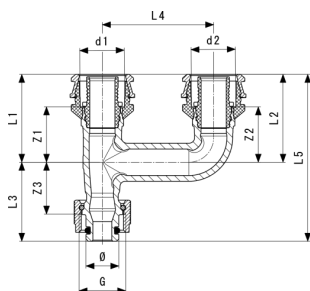
Raxofix-Erweiterungsstück - Siliziumbronze Modell 5325.78
