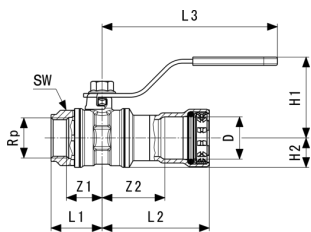
Megapress G-Gaskugelhahn - Stahl unlegiert, Zink-Nickel-Beschichtung Modell 4675.4
