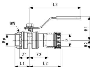
Megapress G-Gaskugelhahn - Stahl unlegiert, Zink-Nickel-Beschichtung Modell 4675.4
