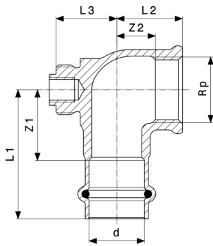
Profipress G-Anschlusswinkel 90° - Rotguss Modell 2614.6
