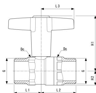
Vanne à bille Easytop modèle 2275.1
