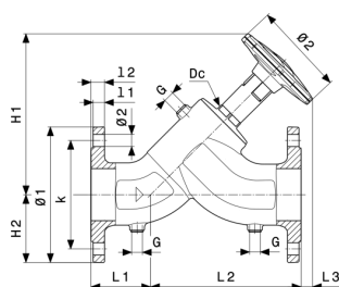
Vanne à siège incliné Easytop XL modèle 2238.5XL
