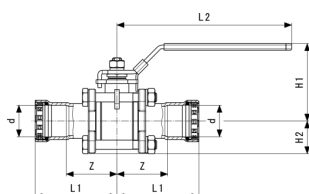
Vanne à bille Easytop XL - acier non allié, revêtement zinc-nickel modèle 4275.8XL
