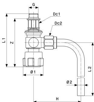
Vanne de prélèvement Easytop modèle 2223.1
