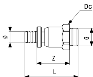
Vanne de vidange Easytop - bronze modèle 2278.7
