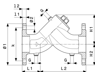
Clapet anti-retour Easytop XL modèle 2239.4XL
