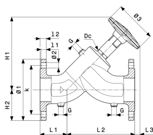
Vanne à siège incliné Easytop XL modèle 2237.5XL
