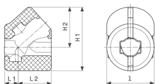
Coque isolante Easytop modèle 2210.35
