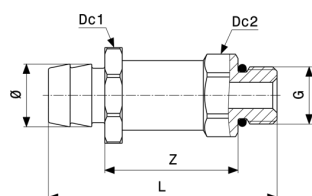
Vanne de vidange Easytop - laiton modèle 2278.8
