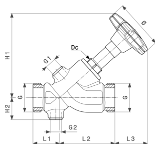
Vanne à siège incliné Easytop modèle 2238.3
