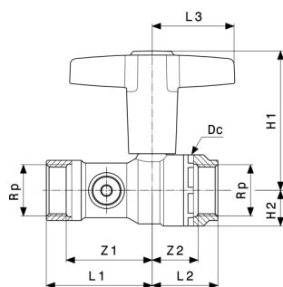
Vanne à bille Easytop modèle 2275.5
