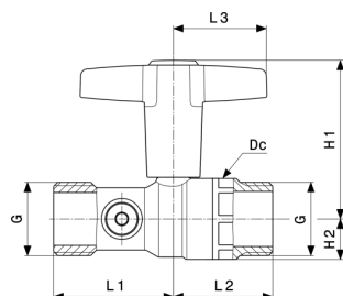
Vanne à bille Easytop modèle 2275.6
