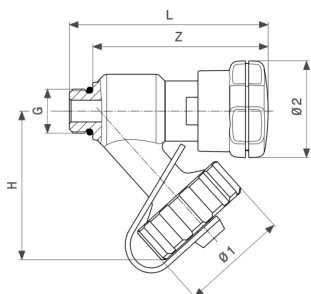
Vanne de vidange Easytop modèle 2234
