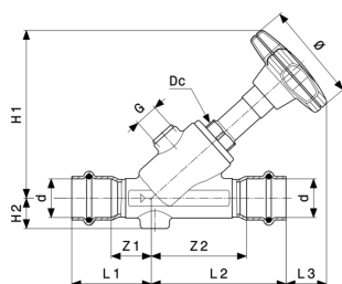
Vanne à siège incliné Easytop Inox - acier inoxydable modèle 2337.5
