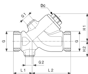
Clapet anti-retour Easytop modèle 2239.3
