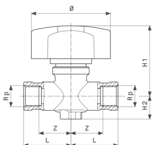
Vanne à flux libre Easytop modèle 2278.1
