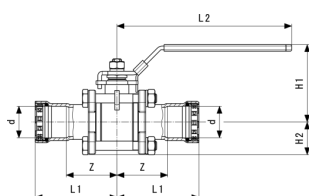
Vanne à bille Easytop - acier non allié, revêtement zinc-nickel modèle 4375.8
