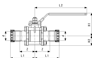
Vanne à bille Easytop - acier non allié, revêtement zinc-nickel modèle 4275.8
