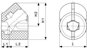
Coque isolante Easytop modèle 2210.12
