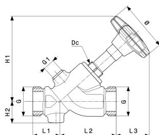
Vanne à siège incliné Easytop modèle 2237.3
