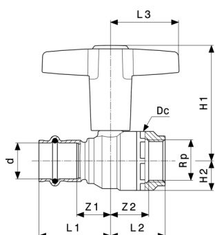
Vanne à bille Easytop modèle 2275.4
