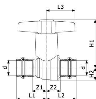
Vanne à bille Easytop - bronze au silicium modèle 2275CO
