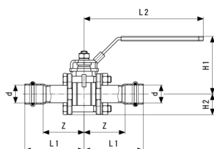
Vanne à bille Easytop - acier inoxydable modèle 2375.8
