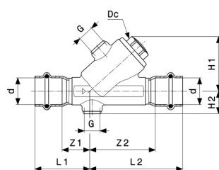
Clapet anti-retour Easytop Inox - acier inoxydable modèle 2339.4
