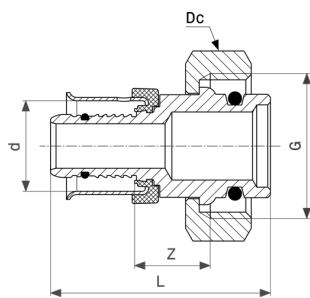
Raccord fileté Pexfit Pro - bronze modèle 4722P
