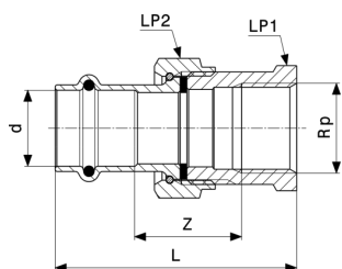
Profipress S-Raccord démontable de transition - bronze ou bronze au silicium modèle 4562
