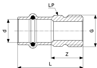
Profipress S-Pièce de transition - bronze ou bronze au silicium modèle 4511.4
