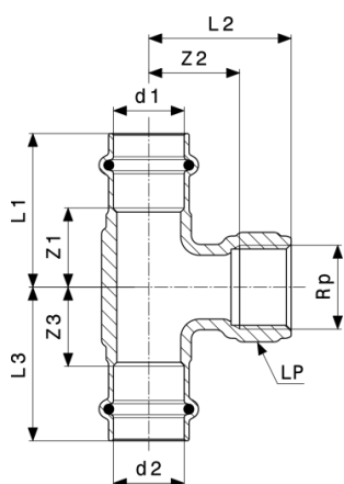
Profipress S-Té - bronze ou bronze au silicium modèle 4517.2
