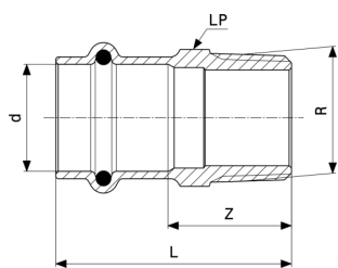
Profipress S-Pièce de transition - bronze ou bronze au silicium modèle 4511
