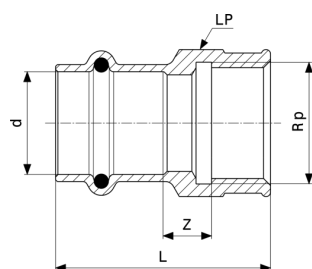
Profipress S-Pièce de transition - bronze ou bronze au silicium modèle 4512
