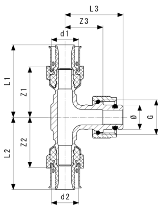
Viega Smartpress-Té transitaire - bronze modèle 6718.8
