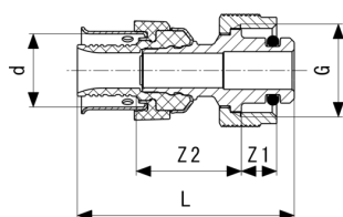
Viega Smartpress-Pièce de transition - bronze modèle 6711.8
