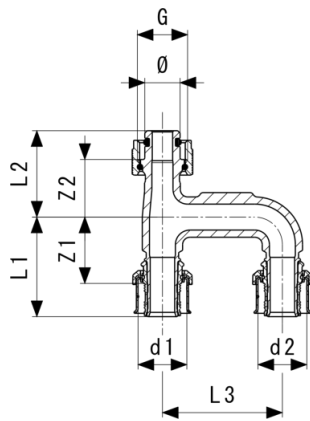
Viega Smartpress-Pièce d'extension - bronze modèle 6725.78
