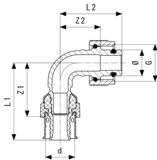
Viega Smartpress-Coude de transition 90° - bronze modèle 6716.8
