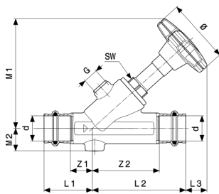
Easytop ferde ülésű szelep modellszám 2237.5
