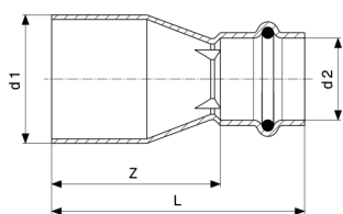
Profipress szűkítődíom - vörösréz modellszám 2415.1
