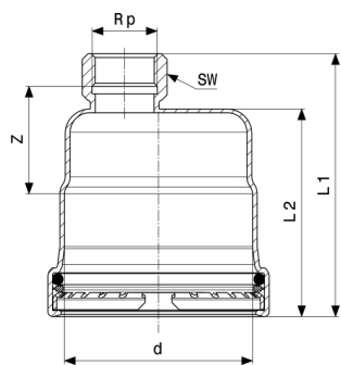
Profipress XL zárókupak - vörösréz modellszám 2456XL
