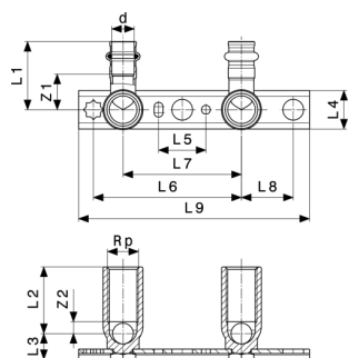
Sanpress szerelőegység modellszám 2221.1
