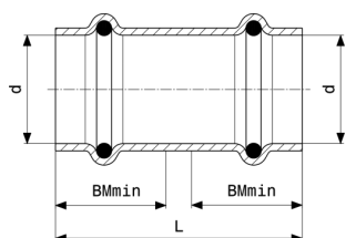
Profipress áttolóarmantyú - vörösréz modellszám 2415.3
