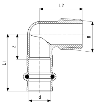
Sanpress 90°-os átmenőkönyök - vörösöntvény vagy szilíciumbronz modellszám 2214.1
