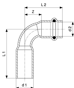
Profipress 90°-os szűkítőív - vörösréz modellszám 2416.2
