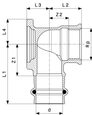
Sanpress falikorong - vörösöntvény vagy szilíciumbronz modellszám 2225.5
