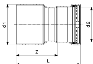
Profipress XL szűkítődíom - vörösréz modellszám 2415.1XL
