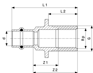
Sanpress falátvezető - vörösöntvény vagy szilíciumbronz modellszám 2232.3
