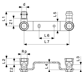
Sanpress szerelőegység modellszám 2222.6EX
