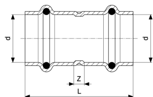
Profipress karmantyú - vörösréz modellszám 2415
