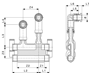
Padlószegélybe építhető fűtőtest-csatlakozó - vörösöntvény modellszám 2277.2
