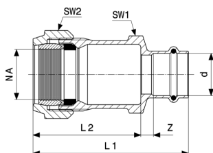
Sanpress átmenőcsavarzat - vörösöntvény vagy szilíciumbronz modellszám 2215.6
