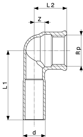
Sanpress bedugós könyök 90° - vörösöntvény vagy szilíciumbronz modellszám 2214.3
