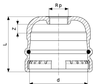
Sanpress XL zárókupak - vörösöntvény modellszám 2256XL
