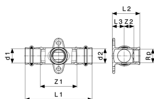
Sanpress falikorong T-idom - vörösöntvény vagy szilíciumbronz modellszám 2217.3
