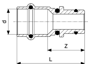
Sanpress bedugós adapter - vörösöntvény modellszám 2233.5
