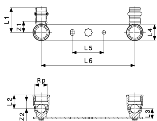
Sanpress szerelőegység modellszám 2222.05
