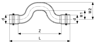
Profipress kerülőív - vörösréz modellszám 2428
