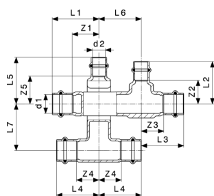
Sanpress keresztező T-idom - vörösöntvény modellszám 2249.3
