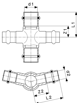
Sanpress 24°-os keresztező idom - vörösöntvény modellszám 2247
