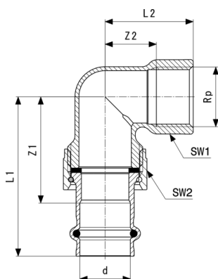
Sanpress átmenőcsavarzat 90° - vörösöntvény vagy szilíciumbronz modellszám 2255
