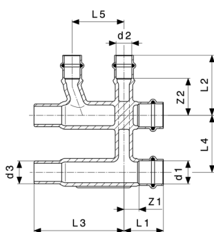
Sanpress esztrich-osztó - vörösöntvény modellszám 2252
