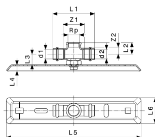
Sanpress szerelőegység modellszám 2218.4
