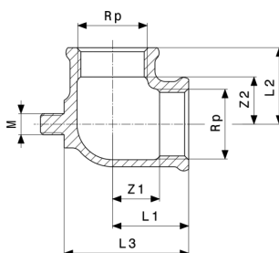
90°-os csatlakozókönyök - vörösöntvény vagy szilíciumbronz modellszám 94477.0-713
