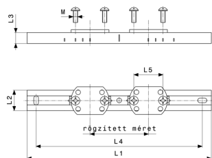
Tartó - horganyzott acél modellszám 2141.3
