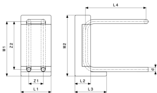
Fűtőtest-csatlakozóblokk modellszám 1097.6
