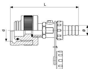
Nyomáspróbádugó - sárgaréz modellszám 2269
