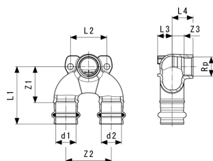
Sanpress kettős falikorong - vörösöntvény vagy szilíciumbronz modellszám 2228.7
