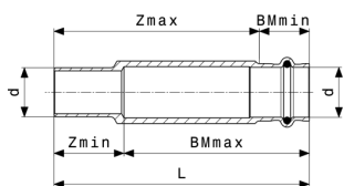
Sanpress áttolókarmantyú - vörösöntvény vagy szilíciumbronz modellszám 2215.4
