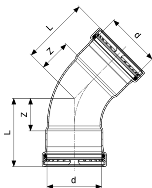
Profipress XL 45°-os ív - vörösréz modellszám 2426XL
