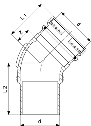
Sanpress XL 45°-os ív - vörösöntvény modellszám 2226.1XL
