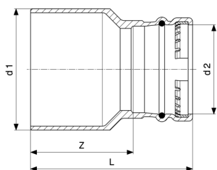
Sanpress XL szűkítőidom - vörösöntvény modellszám 2215.1XL
