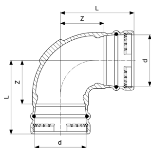
Sanpress XL 90°-os ív - vörösöntvény modellszám 2216XL
