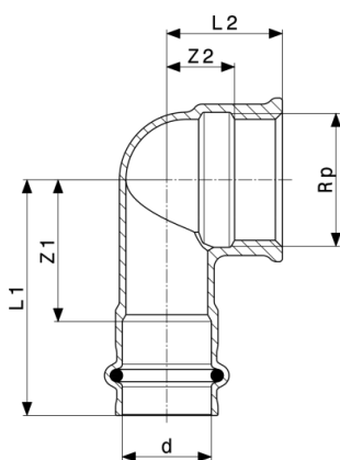
Sanpress 90°-os átmenőkönyök - vörösöntvény vagy szilíciumbronz modellszám 2214.2
