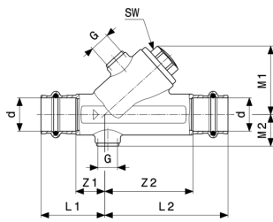
Easytop visszacsapó szelep modellszám 2239.4
