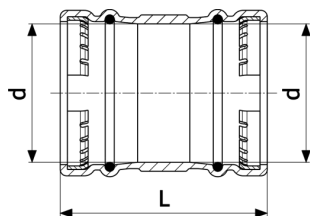
Sanpress XL áttolóarmantyú - vörösöntvény modellszám 2215.5XL
