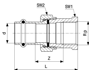
Sanpress átmenőcsavarzat - vörösöntvény vagy szilíciumbronz modellszám 2262
