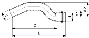
Profipress kerülőív - vörösréz modellszám 2427
