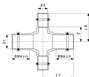
Sanpress keresztező idom - vörösöntvény vagy szilíciumbronz modellszám 2244
