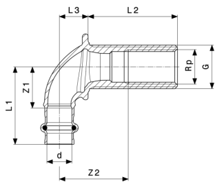
Sanpress falátvezető - vörösöntvény vagy szilíciumbronz modellszám 2232.1
