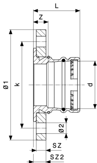
Sanpress XL karimás átmeneti idom - vörösöntvény modellszám 2259.5XL
