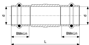
Sanpress áttolókarmantyú - vörösöntvény vagy szilíciumbronz modellszám 2215.5
