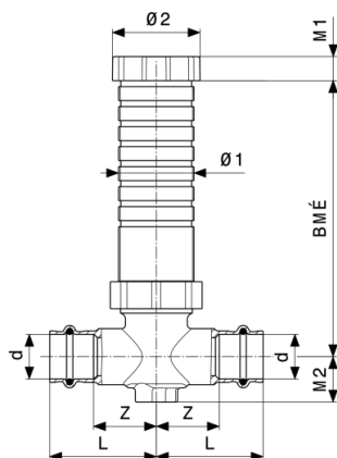
Easytop vakolat alatti csempeszelep modellszám 2278.5
