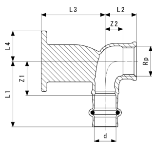
Sanpress falikorong - vörösöntvény vagy szilíciumbronz modellszám 2225.6
