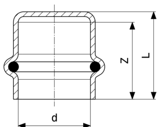
Profipress zárókupak - vörösréz modellszám 2456
