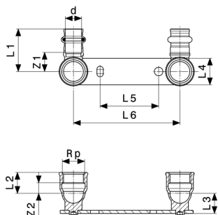
Sanpress szerelőegység modellszám 2222.2
