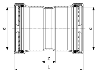
Profipress XL karmantyú - vörösréz modellszám 2415XL
