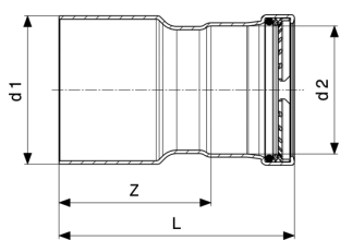
Profipress XL szűkítőidom - vörösréz modellszám 2415.1XL
