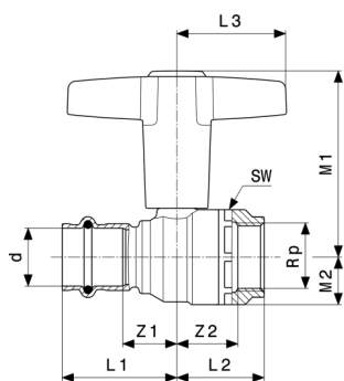
Easytop gömbcsap modellszám 2275.4
