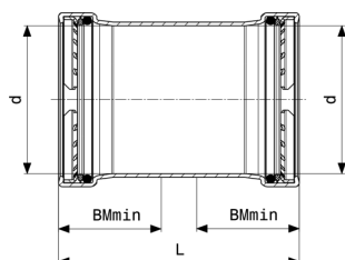
Profipress XL áttolóarmantyú - vörösréz modellszám 2415.5XL
