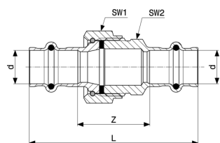
Sanpress csavarzat - vörösöntvény vagy szilíciumbronz modellszám 2260
