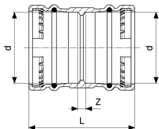
Sanpress XL karmantyú - vörösöntvény modellszám 2215XL
