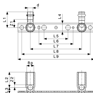
Sanpress szerelőegység modellszám 2221
