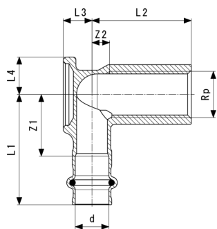
Sanpress falikorong - vörösöntvény vagy szilíciumbronz modellszám 2225
