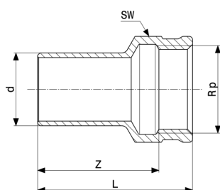
Sanpress bedugóidom - vörösöntvény vagy szilíciumbronz modellszám 2212.1
