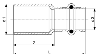
Sanpress szűkítőidom - vörösöntvény vagy szilíciumbronz modellszám 2215.1
