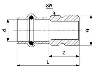
Sanpress átmeneti idom - vörösöntvény vagy szilíciumbronz modellszám 2211.4
