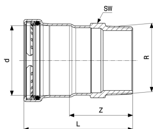
Profipress XL átmeneti idom - vörösréz modellszám 2411XL
