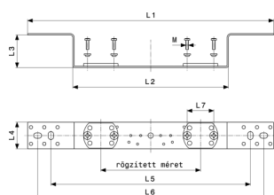
Tartó - horganyzott acél modellszám 2021.7
