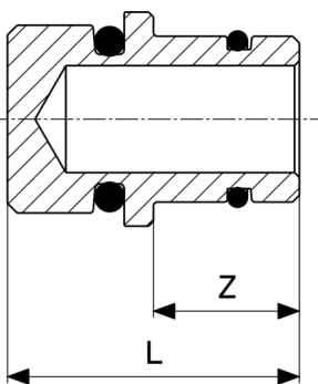
Bedugós adapter - vörösöntvény vagy szilíciumbronz modellszám 2233.6
