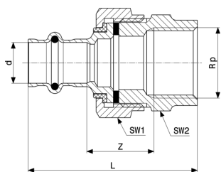
Sanpress szigetelő csavarzat - vörösöntvény vagy szilíciumbronz modellszám 2267
