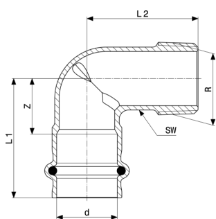
Sanpress 90°-os átmenőív - vörösöntvény vagy szilíciumbronz modellszám 2214
