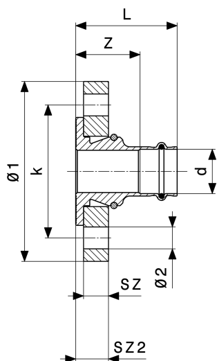
Sanpress karimás átmeneti idom - vörösöntvény vagy szilíciumbronz modellszám 2259.5
