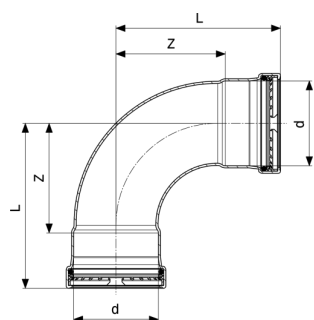
Profipress XL 90°-os ív - vörösréz modellszám 2416XL
