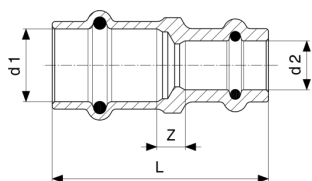
Sanpress szűkítőkarmantyú - vörösöntvény modellszám 9778.0
