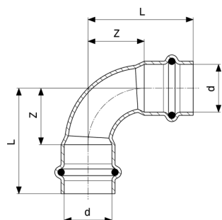
Profipress 90°-os ív - vörösréz modellszám 2416
