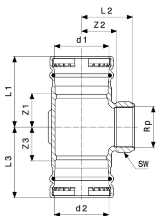
Sanpress XL T-idom - vörösöntvény modellszám 2217.2XL
