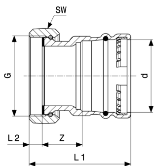
Sanpress XL csatlakozócsavarzat - vörösöntvény modellszám 2263XL
