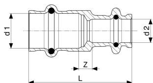
Sanpress szűkítőkarmantyú - vörösöntvény modellszám 9778.1
