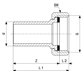
Sanpress csatlakozócsavarzat - vörösöntvény vagy szilíciumbronz modellszám 2264
