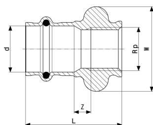
Sanpress átmeneti idom - vörösöntvény vagy szilíciumbronz modellszám 2212.3
