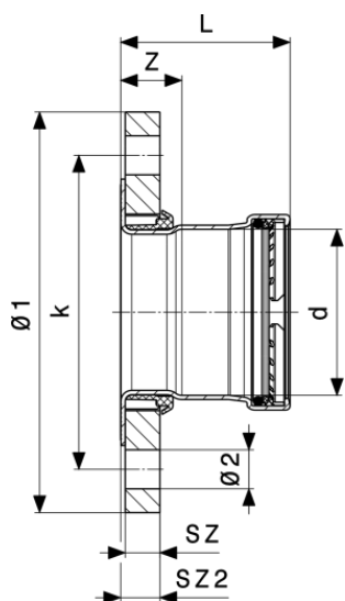
Profipress XL karimás átmeneti idom - vörösréz modellszám 2459.5XL
