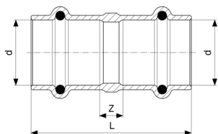
Sanpress karmantyú - vörösöntvény modellszám 9777.9
