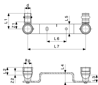
Sanpress szerelőegység modellszám 2222
