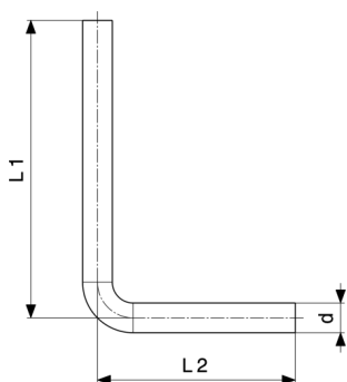
90°-os csatlakozóív - nemesacél modellszám 2271.1
