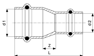
Profipress szűkítőkarmantyú - vörösréz modellszám 2415.2
