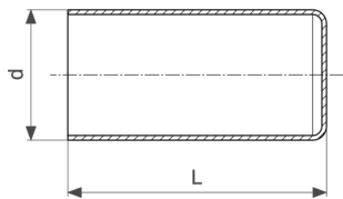
Prestabo záródugó - ötvöztelen, horganyzott acél modellszám 1157.1
