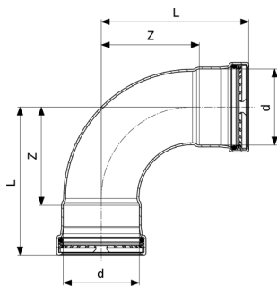
Prestabo XL 90°-os ív - ötvözetlen, horganyzott acél modellszám 1116XL
