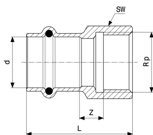
Prestabo átmeneti idom - ötvözetlen, horganyzott acél modellszám 1112
