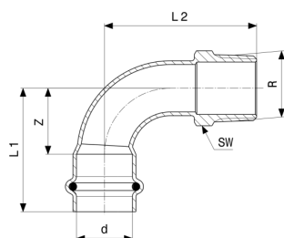
Prestabo 90°-os átmenőív - ötvözetlen, horganyzott acél modellszám 1114
