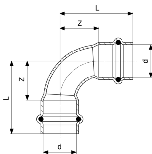
Prestabo 90°-os ív - ötvözetlen, horganyzott acél modellszám 1116
