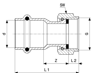
Prestabo csatlakozócsavarzat - ötvöztelen, horganyzott acél modellszám 1163
