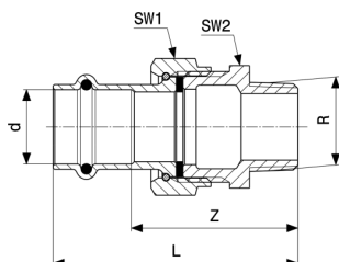
Prestabo átmenőcsavarzat - ötvözetlen, horganyzott acél modellszám 1165
