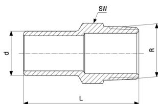
Prestabo bedugóidom - ötvözetlen, horganyzott acél modellszám 1111.1
