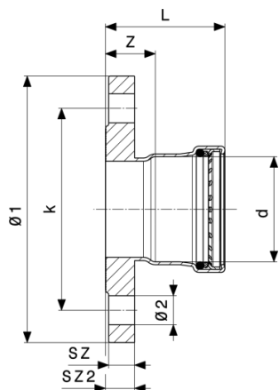
Prestabo XL karimás átmeneti idom - ötvözetlen, horganyzott acél modellszám 1159.1XL
