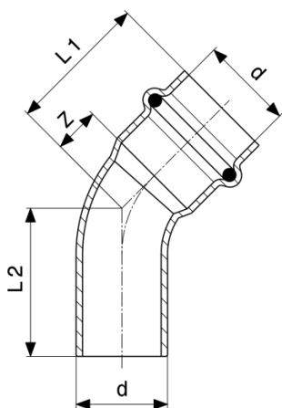
Prestabo 45°-os ív - ötvöztelen, horganyzott acél modellszám 1126.1
