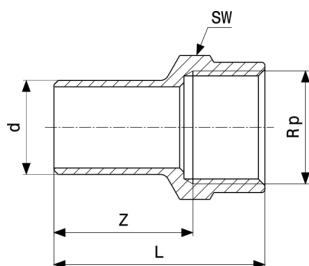
Prestabo bedugóidom - ötvözetlen, horganyzott acél modellszám 1112.1
