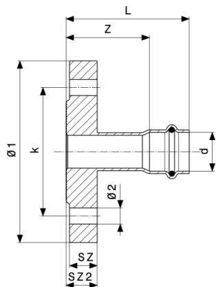
Prestabo karimás átmeneti idom - ötvözetlen, horganyzott acél modellszám 1159
