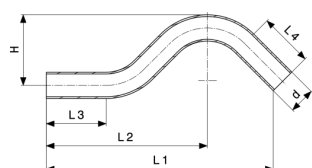
Prestabo kerülőív - ötvözetlen, horganyzott acél modellszám 1109.3
