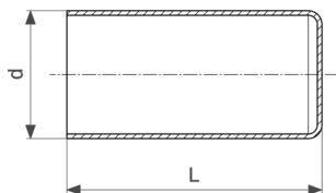
Prestabo XL záródugó - ötvözetlen, horganyzott acél modellszám 1157.1XL
