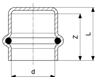
Prestabo zárókupak - ötvöztelen, horganyzott acél modellszám 1156
