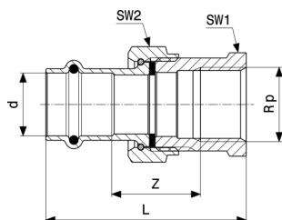
Prestabo átmenőcsavarzat - ötvözetlen, horganyzott acél modellszám 1162
