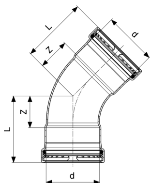
Prestabo XL 45°-os ív - ötvöztelen, horganyzott acél modellszám 1126XL
