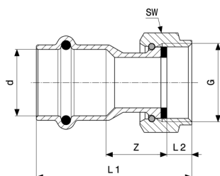
Prestabo csatlakozócsavarzat - ötvözetlen, horganyzott acél modellszám 1163
