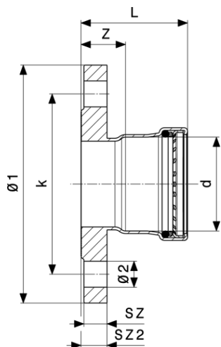
Prestabo XL karimás átmeneti idom - ötvözetlen, horganyzott acél modellszám 1159XL
