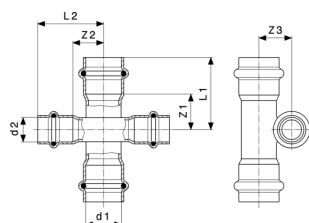
Prestabo keresztező idom - ötvözetlen, horganyzott acél modellszám 1148
