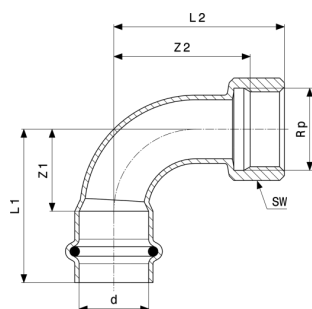
Prestabo 90°-os átmenőív - ötvözetlen, horganyzott acél modellszám 1114.5
