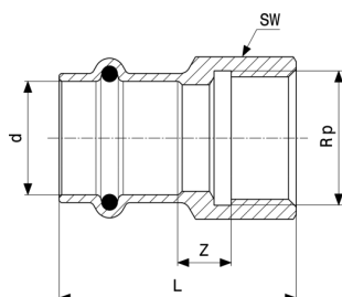
Prestabo átmeneti idom - ötvözetlen, horganyzott acél modellszám 1112
