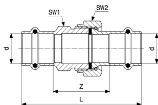
Prestabo csavarzat - ötvözetlen, horganyzott acél modellszám 1160
