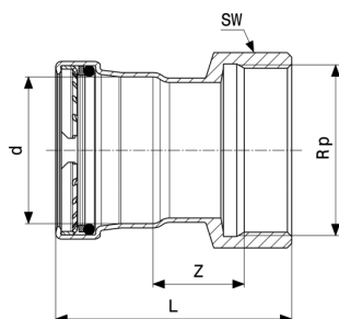
Prestabo XL átmeneti idom - ötvözetlen, horganyzott acél modellszám 1112XL
