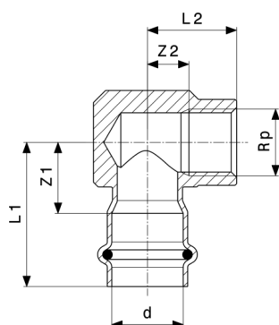
Prestabo 90°-os átmenőkönyök - ötvözetlen, horganyzott acél modellszám 1114.2
