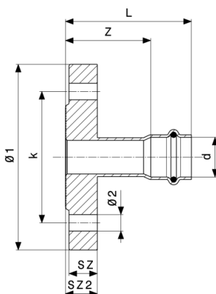
Prestabo karimás átmeneti idom - ötvözetlen, horganyzott acél modellszám 1159.1
