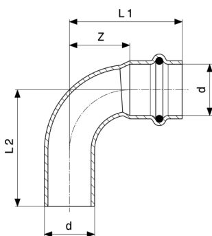
Prestabo 90°-os ív - ötvözetlen, horganyzott acél modellszám 1116.1
