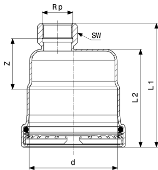
Prestabo XL zárókupak - ötvöztelen, horganyzott acél modellszám 1156XL
