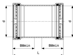
Prestabo XL áttolóarmantyú - ötvözetlen, horganyzott acél modellszám 1115.5XL
