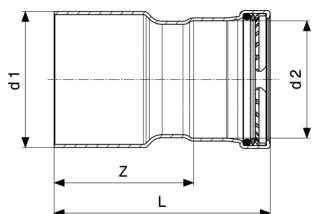
Prestabo XL szűkítőidom - ötvözetlen, horganyzott acél modellszám 1115.1XL
