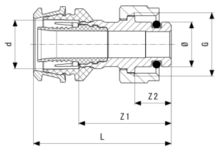
Manicotto Raxofix - bronzo al silicio Modello 5311.8
