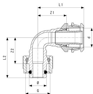
Curva a 90° Raxofix - bronzo al silicio Modello 5316.8
