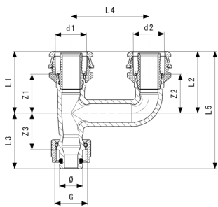
Raccordo doppio Raxofix - bronzo al silicio Modello 5325.78
