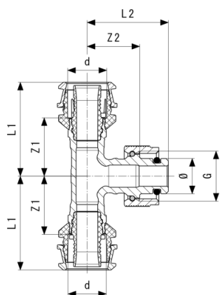
Raccordo a T di passaggio Raxofix - bronzo al silicio Modello 5318.8
