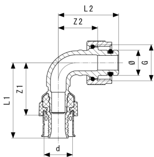
Curva a 90° Viega Smartpress - bronzo Modello 6716.8
