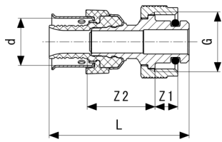
Manicotto Viega Smartpress - bronzo Modello 6711.8
