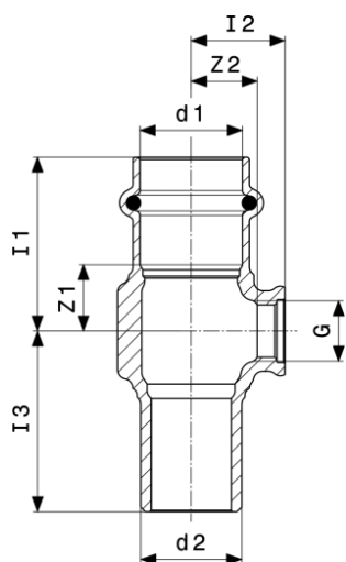
Sanpress-triřakis - raudonoji bronza arba silicio bronza modelis 2217.4
