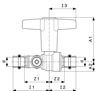
Easytop-rutulinis čiaupas modelis 2275.3
