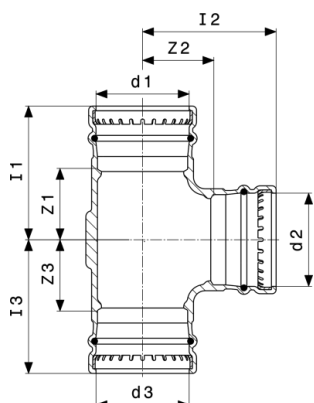
Sanpress XL-triškis - raudonoji bronza modelis 2218XL
