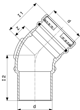
Sanpress XL-alkūnē 45° - raudonoji bronza modelis 2226.1XL
