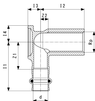
Sanpress-tvirtinamai detalei - raudonoji bronzą arba silicio bronzą modelis 2225
