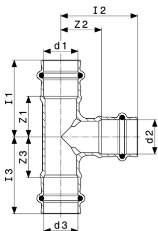
Sanpress-triškis - raudonoji bronza arba silicio bronza modelis 2218
