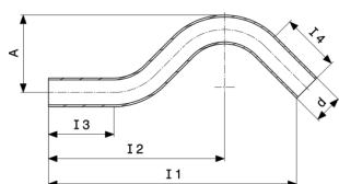
Sanpress-apejimas - nerūdijantis plienas modelis 2209.3
