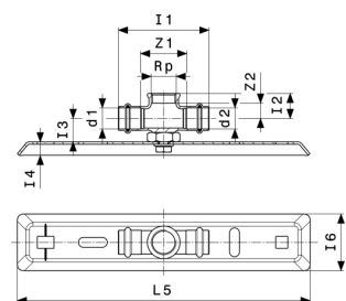
Sanpress-montavimo blokas modelis 2218.4
