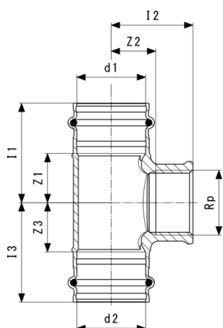
Sanpress-triškakis - raudonoji bronzos arba silicio bronzos modelis 2217.2
