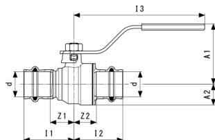
Easytop-rutulinis čiaupas - silicio bronza modelis 2275.10
