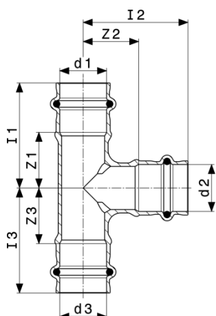
Sanpress-triškakis - raudonoji bronza arba silicio bronza modelis 2218
