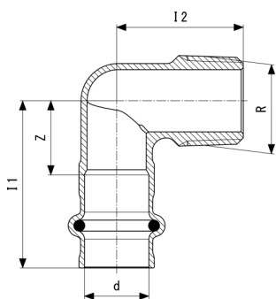
Sanpress-pereinamoji alkūnė 90° - raudonoji bronza arba silicio bronza modelis 2214.1
