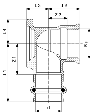
Sanpress-tvirtinamai detalei - raudonoji bronzą arba silicio bronzą modelis 2225.5
