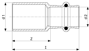
Sanpress-mova - raudonoji bronza arba silicio bronza modelis 2215
