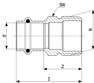
Sanpress-pereinamoji detalė - raudonoji bronza arba silicio bronza modelis 2211
