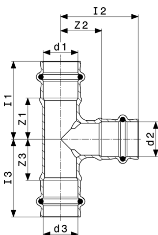
Sanpress-trišakis - raudonoji bronza arba silicio bronza modelis 2218
