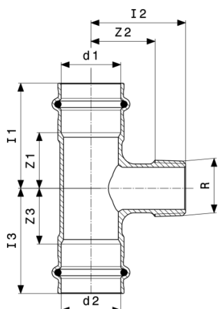
Sanpress-triškakis - raudonoji bronza arba silicio bronza modelis 2217.1
