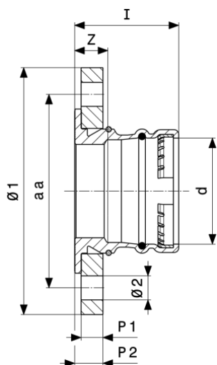
Sanpress XL-flanšo pereiga - raudonoji bronza modelis 2259.3XL
