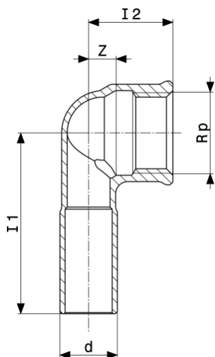
Sanpress-įkišama alkūnė 90° - raudonoji bronzą arba silicio bronzą modelis 2214.3
