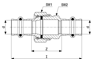
Sanpress-srieginė jungtis - raudonoji bronzė arba silicio bronzė modelis 2260
