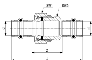
Sanpress-srieginė jungtis - raudonoji bronzė arba silicio bronzė modelis 2260
