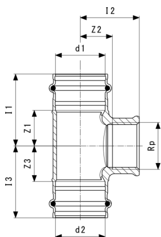
Sanpress-triškakis - raudonoji bronza arba silicio bronza modelis 2217.2
