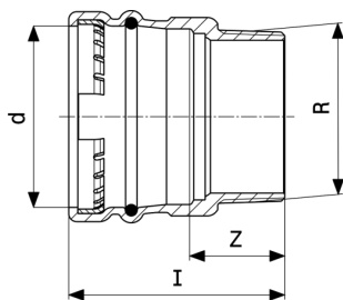
Sanpress XL-pereinamoji detalė - raudonoji bronza modelis 2211XL
