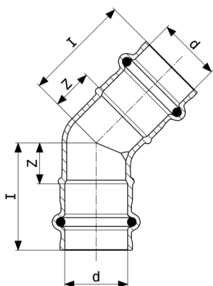
Sanpress-alkūnē 45° - raudonoji bronza arba silicio bronza modelis 2226
