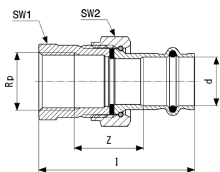
Sanpress-pereinamoji srieginė jungtis - raudonoji bronzė arba silicio bronzė modelis 2262
