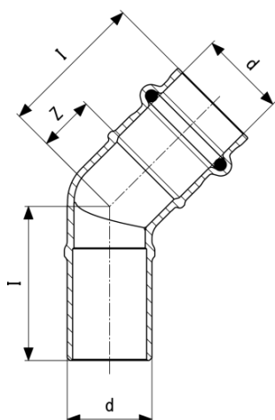
Sanpress-alkūnē 45° - raudonoji bronza arba silicio bronza modelis 2226.1
