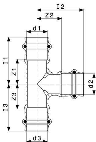
Sanpress-triškakis - raudonoji bronza arba silicio bronza modelis 2218
