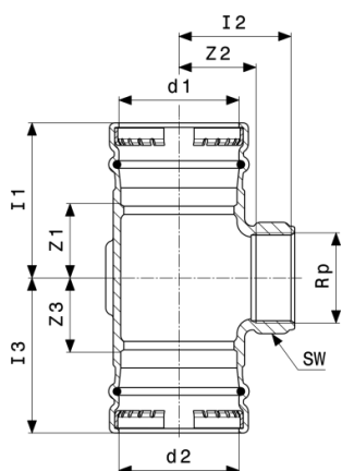
Sanpress XL-triškakis - raudonoji bronza modelis 2217.2XL
