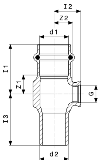
Sanpress-triškakis - raudonoji bronza arba silicio bronza modelis 2217.4
