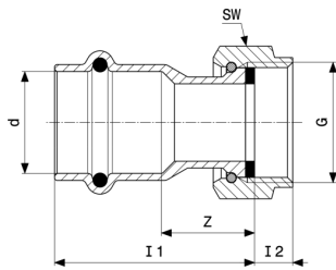
Sanpress-jungiamoji srieginė jungtis - raudonoji bronzė arba silicio bronzė modelis 2263
