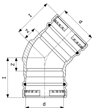
Sanpress XL-alkūnē 45° - raudonoji bronza modelis 2226XL
