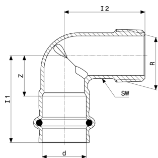
Sanpress-pereinamoji alkūnė 90° - raudonoji bronzą arba silicio bronzą modelis 2214
