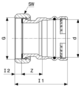
Sanpress XL-jungiamoji srieginė jungtis - raudonoji bronza modelis 2263XL
