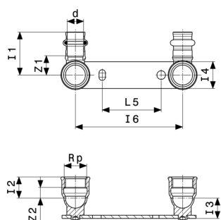
Sanpress-montavimo blokas modelis 2222.2
