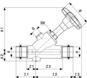
Easytop-įstrižinis vožtuvas modelis 2237.5
