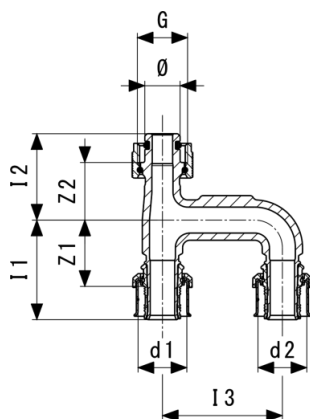
Viega Smartpress-praplėtimo detalė - raudonoji bronzą modelis 6725.78
