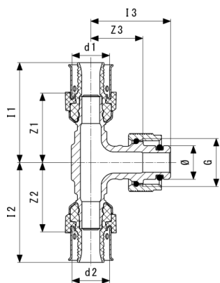
Viega Smartpress-triřakis - raudonoji bronza modelis 6718.8
