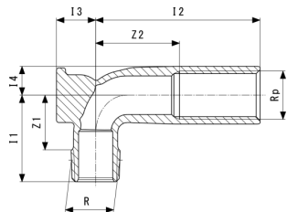
Tvirtinama detalė, skirta „Prevista“ - silicio bronza modelis 8055.2
