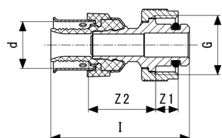
Viega Smartpress-pereinamoji detalė - raudonoji bronza modelis 6711.8
