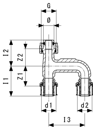
Viega Smartpress-praplétimo detalė - raudonoji bronza modelis 6725.78
