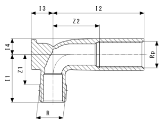
Tvirtinama detalė, skirta „Prevista“ - silicio bronza modelis 8055.2
