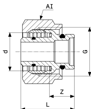
Spīlgredzena skrūšsavienojums - misiņš modelis 1019
