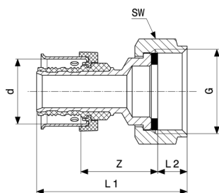
Viega Smartpress schroefkoppeling - brons model 6763
