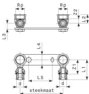
Viega Smartpress montage-unit - staal verzinkt model 6724.2
