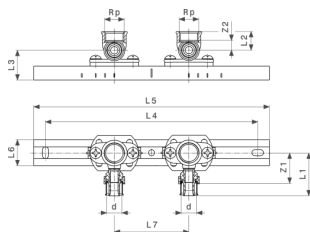
Viega Smartpress montage-unit - staal verzinkt model 6741
