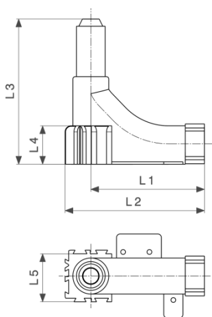
Buisgeleidingsbocht 90° model 1072.3
