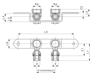
Viega Smartpress montage-unit - staal verzinkt model 6723.1
