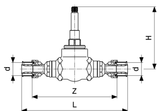
Viega Smartpress inbouw-vrijstroomventiel - messing model 6770
