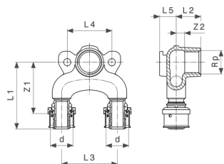
Viega Smartpress doorstroommuurplaat - brons model 6725.7
