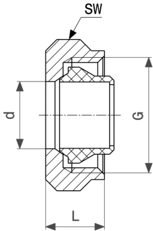
Schroefkoppeling - messing vernikkeld model 94385.2
