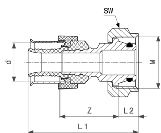
Viega Smartpress schroefkoppeling - brons model 6783
