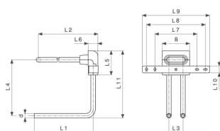
Viega Smartpress radiatoraansluitblok - meerlagenbuis model 6797.7
