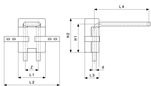
Radiatoraansluitblok model 1097.9
