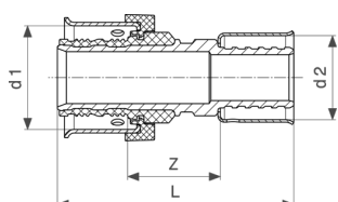
Viega Smartpress G overgangsstukkoppeling - brons model 6715G
