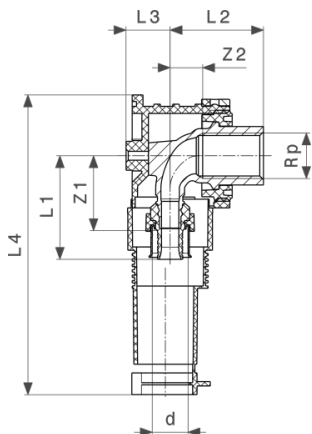
Viega Smartpress aansluitdoos 90° - brons model 6720.01
