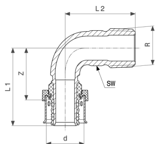
Viega Smartpress overgangstukbocht 90° - brons model 6714
