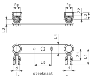
Viega Smartpress montage-unit - staal verzinkt model 6724.1
