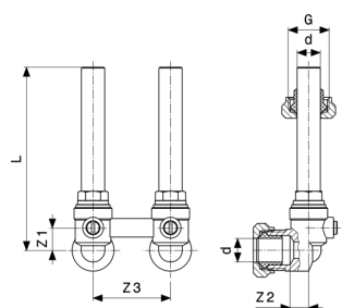
Radiatoraansluitset - messing met vernikkeld model 1097.7
