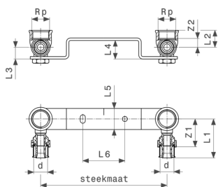
Viega Smartpress montage-unit - staal verzinkt model 6724
