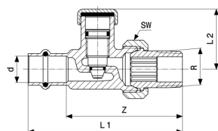
Sanpress retourventiel - brons model 2272.2
