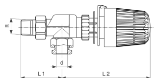
Haaksverkeerde radiatorkraan - messing vernikkeld model 1075.96
