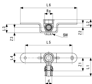
Viega Smartpress montage-unit - staal verzinkt model 6723
