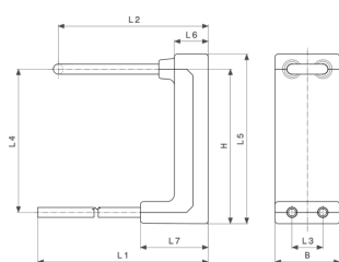
Viega Smartpress radiatoraansluitblok - meerlagenbuis model 6797.6
