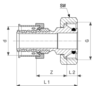
Viega Smartpress schroefkoppeling - brons model 6735
