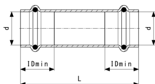
Temponox schuifsok - roestvast staal model 1715.5
