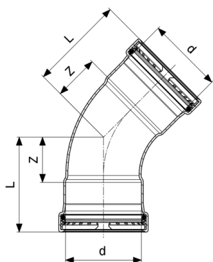
Temponox XL bocht 45° - roestvast staal model 1726XL
