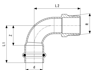
Temponox overgangstukbocht 90° - roestvast staal model 1714
