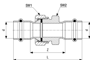
Temponox schroefkoppeling - roestvast staal model 1760
