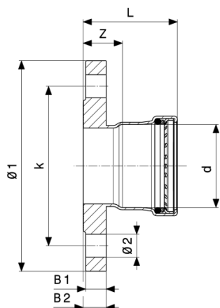
Temponox XL flensovergangsstuk - roestvast staal model 1759.1XL
