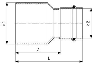
Temponox XL reductiestuk - roestvast staal model 1715.1XL
