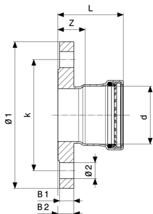
Temponox XL flensovergangsstuk - roestvast staal model 1759XL
