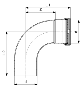
Temponox XL bocht 90° - roestvast staal model 1716.1XL
