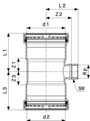
Temponox XL T-stuk - roestvast staal model 1717.2XL
