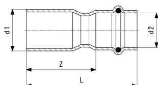
Temponox reductiestuk - roestvast staal model 1715.1
