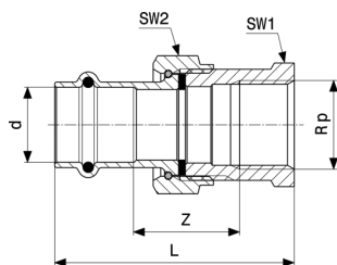
Temponox overgangsschroefkoppeling - roestvast staal model 1762
