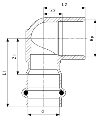
Temponox overgangsstukkie 90° - roestvast staal model 1714.2
