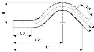
Temponox sprongbochten - roestvast staal model 1709.3
