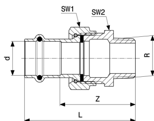
Temponox overgangsschroefkoppeling - roestvast staal model 1765
