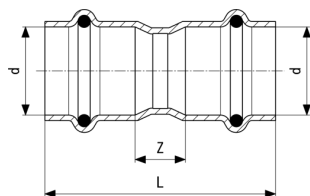
Temponox sok - roestvast staal model 1715
