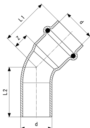
Temponox bocht 45° - roestvast staal model 1726.1
