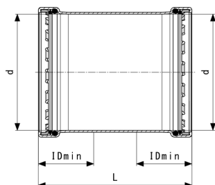
Temponox XL schuifsok - roestvast staal model 1715.5XL
