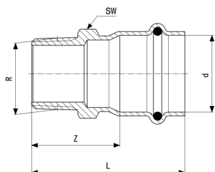
Temponox overgangsstuk - roestvast staal model 1711
