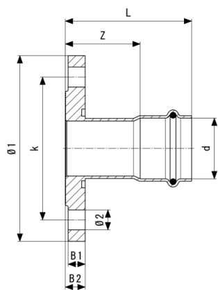
Temponox flensovergangsstuk - roestvast staal model 1759.1
