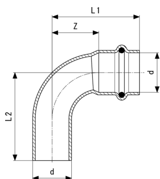
Temponox bocht 90° - roestvast staal model 1716.1
