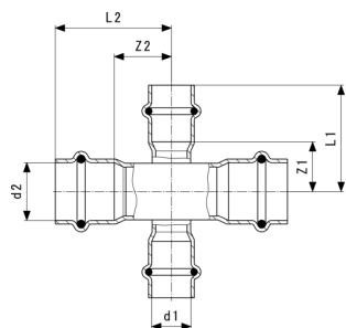
Temponox kruisstuk - roestvast staal model 1748
