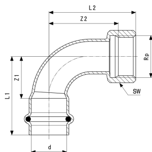
Temponox overgangsstukbocht 90° - roestvast staal model 1714.5
