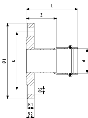
Temponox flensovergangsstuk - roestvast staal model 1759
