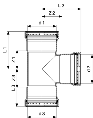
Temponox XL T-stuk - roestvast staal model 1718XL
