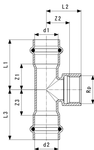
Temponox T-stuk - roestvast staal model 1717.2
