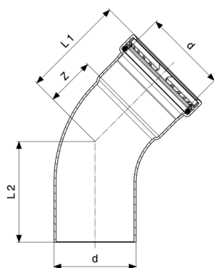
Temponox XL bocht 45° - roestvast staal model 1726.1XL
