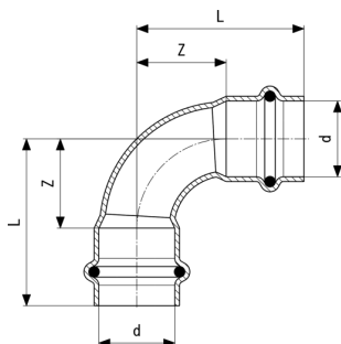
Temponox bocht 90° - roestvast staal model 1716
