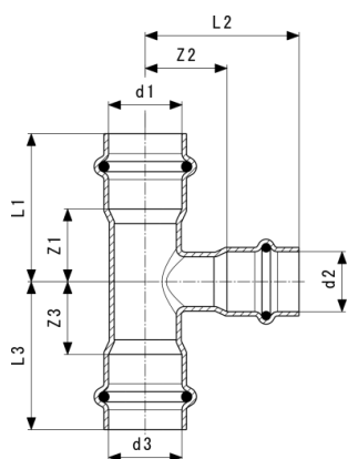
Temponox T-stuk - roestvast staal model 1718
