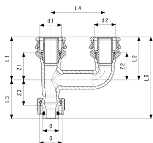
Raxofix-Piesă prelungitoare - bronz siliconic model 5325.78
