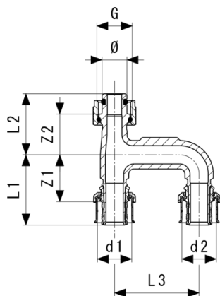
Viega Smartpress-Piesă prelungitoare - bronz model 6725.78
