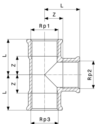
T-kus - mosadz model 1622
