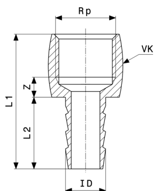
Hadicový nátrubok - mosadz model 1846
