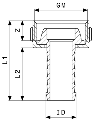
Hadicový skrutkový spoj - mosadz model 1812
