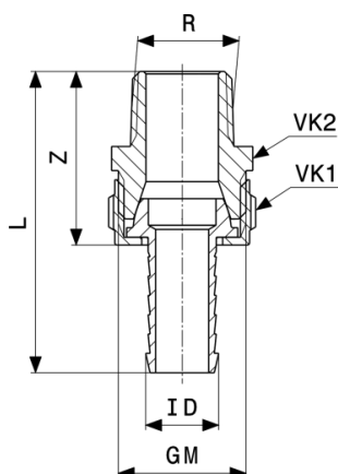
Skrutkový spoj prepadovej rúrky - mosadz model 1832
