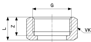
Prevlečná matica - mosadz model 1121-654
