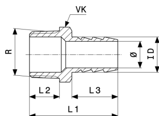
Hadicový nátrubok - mosadz model 1845
