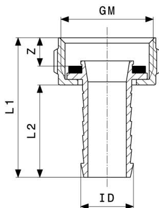
Hadicový skrutkový spoj - mosadz model 1817
