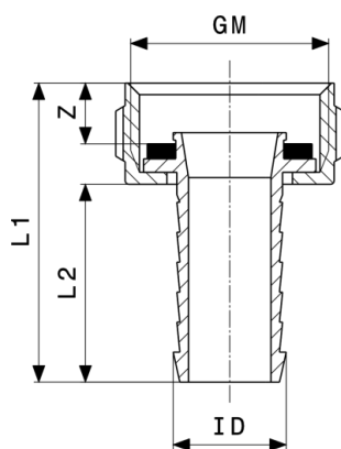
Hadicový skrutkový spoj - mosadz model 1819
