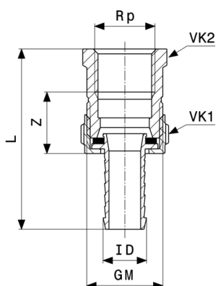
Skrutkový spoj prepadovej rúrky - mosadz model 1841
