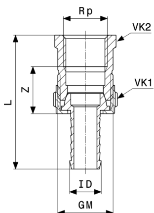
Skrutkový spoj prepadovej rúrky - mosadz model 1842
