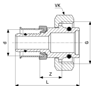
Pexfit Pro-pripájací skrutkový spoj - červený bronz model 4722P
