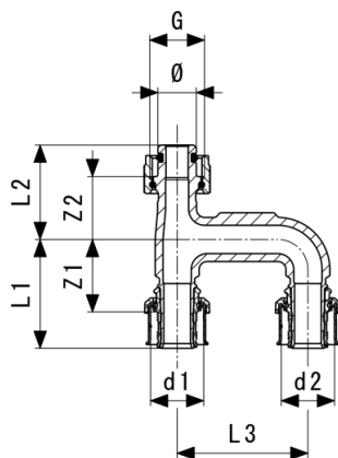
Viega Smartpress-rozširující kus - červený bronz model 6725.78
