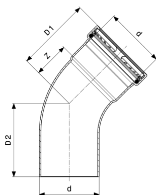
Temponox XL-Lok 45° - nerjavno jeklo Model 1726.1XL
