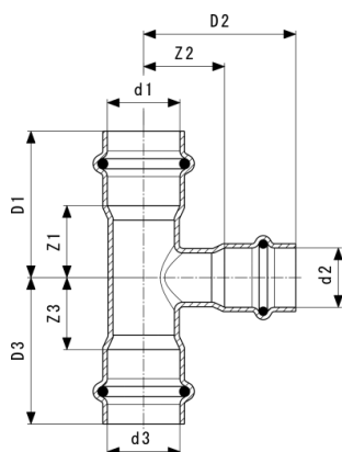
Temponox-T-kos - nerjavno jeklo Model 1718
