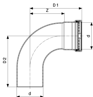
Temponox XL-Lok 90° - nerjavno jeklo Model 1716.1XL
