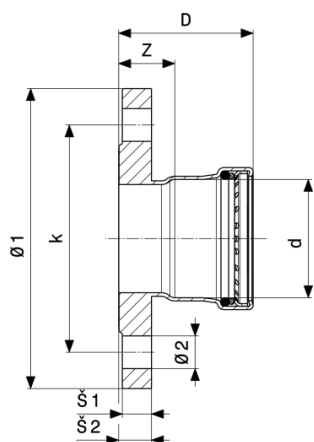
Temponox XL-Prirobnični prehod - nerjavno jeklo Model 1759XL
