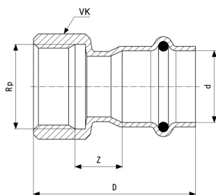
Temponox-Prehodni kos - nerjavno jeklo Model 1712
