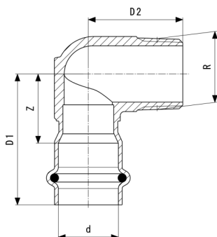
Temponox-Prehodno koleno 90° - nerjavno jeklo Model 1714.1
