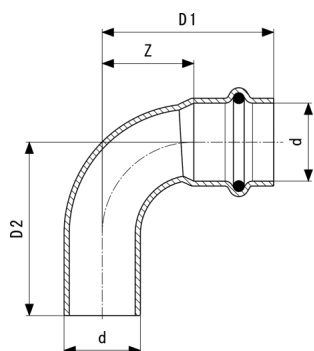
Temponox-Lok 90° - nerjavno jeklo Model 1716.1
