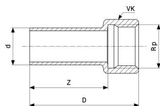
Temponox-Vstavni kos - nerjavno jeklo Model 1712.1
