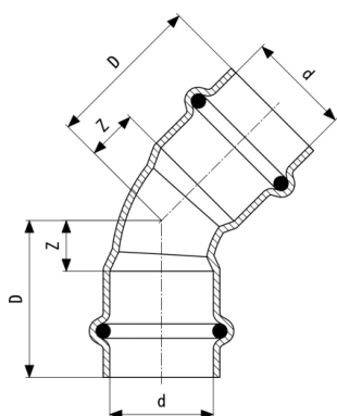
Temponox-Lok 45° - nerjavno jeklo Model 1726
