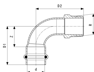
Temponox-Prehodni lok 90° - nerjavno jeklo Model 1714
