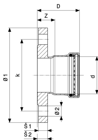
Temponox XL-Prirobnični prehod - nerjavno jeklo Model 1759.1XL
