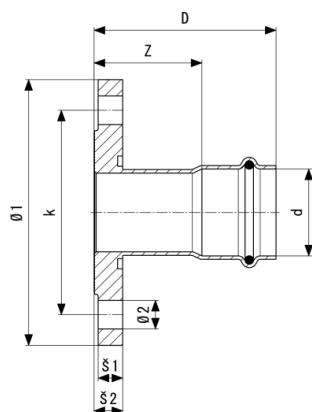
Temponox-Prirobnični prehod - nerjavno jeklo Model 1759.1
