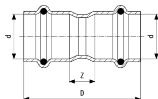
Temponox-Spojka - nerjavno jeklo Model 1715
