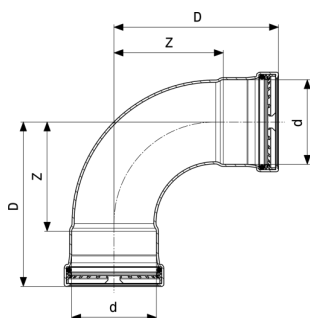
Temponox XL-Lok 90° - nerjavno jeklo Model 1716XL
