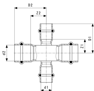
Temponox-Križni kos - nerjavno jeklo Model 1748
