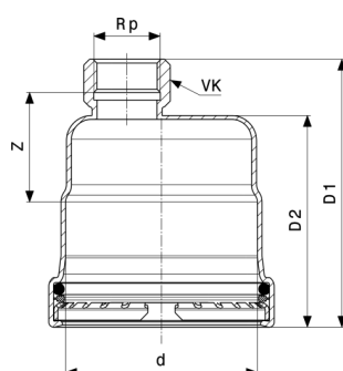
Kapa - nerjavno jeklo Model 1756XL
