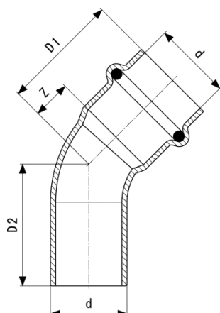
Temponox-Lok 45° - nerjavno jeklo Model 1726.1
