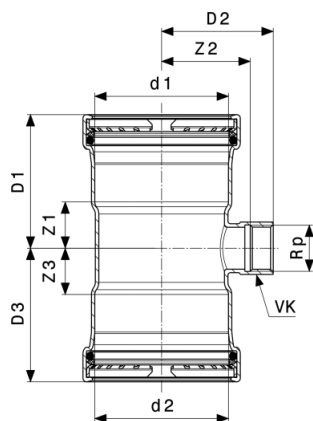
Temponox XL-T-kos - nerjavno jeklo Model 1717.2XL
