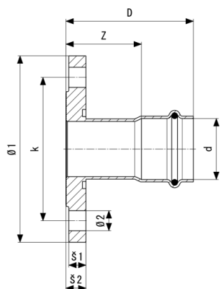
Temponox-Prirobnični prehod - nerjavno jeklo Model 1759
