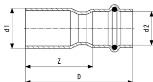
Temponox-Reducirni kos - nerjavno jeklo Model 1715.1
