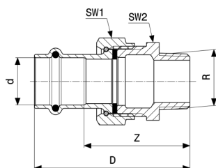
Temponox-Prehodni vijačni spoj - nerjavno jeklo Model 1765
