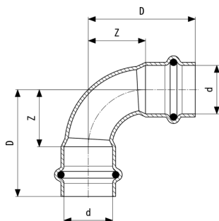
Temponox-Lok 90° - nerjavno jeklo Model 1716
