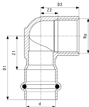
Temponox-Prehodno koleno 90° - nerjavno jeklo Model 1714.2
