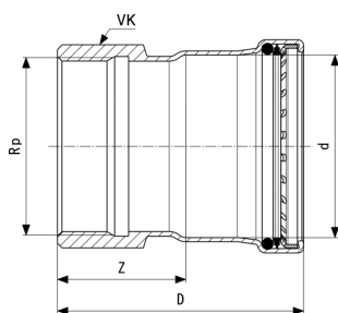
Temponox XL-Prehodni kos - nerjavno jeklo Model 1712XL
