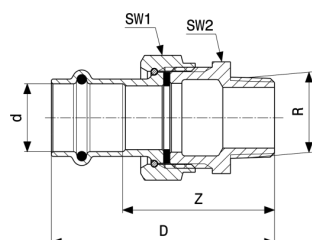
Temponox-Prehodni vijačni spoj - nerjavno jeklo Model 1765
