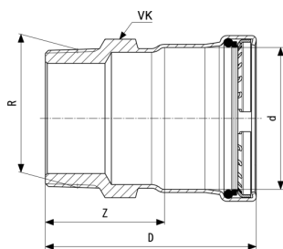
Temponox XL-Prehodni kos - nerjavno jeklo Model 1711XL
