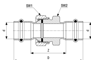
Temponox-Vijačni spoj - nerjavno jeklo Model 1760
