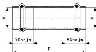
Temponox-Drсна spojka - nerjavno jeklo Model 1715.5
