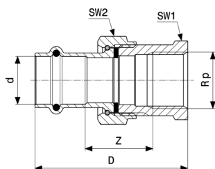
Temponox-Prehodni vijačni spoj - nerjavno jeklo Model 1762
