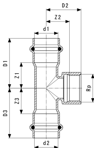
Temponox-T-kos - nerjavno jeklo Model 1717.2
