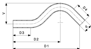
Temponox-Izogibni lok - nerjavno jeklo Model 1709.3
