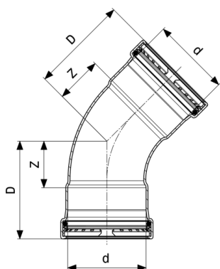
Temponox XL-Lok 45° - nerjavno jeklo Model 1726XL
