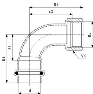
Temponox-Prehodni lok 90° - nerjavno jeklo Model 1714.5
