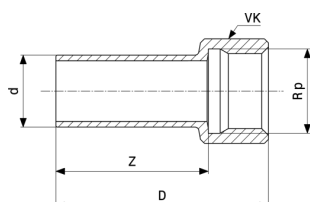
Temponox-Vstavni kos - nerjavno jeklo Model 1712.1
