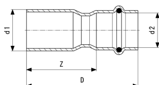
Temponox-Reducirni kos - nerjavno jeklo Model 1715.1
