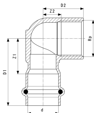
Temponox-Prehodno koleno 90° - nerjavno jeklo Model 1714.2
