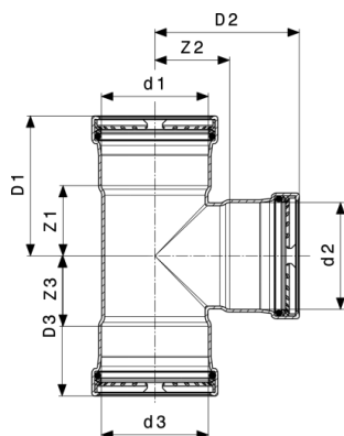
Temponox XL-T-kos - nerjavno jeklo Model 1718XL
