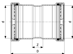
Temponox XL-Spojka - nerjavno jeklo Model 1715XL
