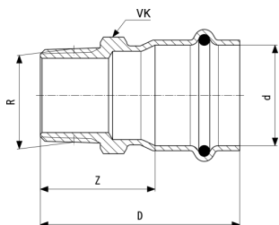
Temponox-Prehodni kos - nerjavno jeklo Model 1711
