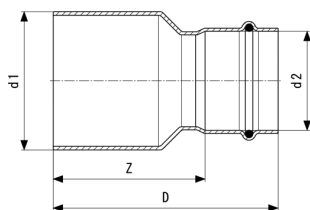
Temponox XL-Reducirni kos - nerjavno jeklo Model 1715.1XL
