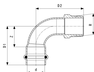
Temponox-Prehodni lok 90° - nerjavno jeklo Model 1714
