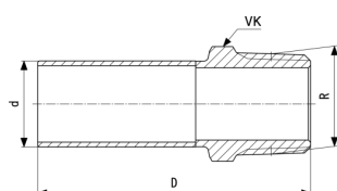
Temponox-Vstavni kos - nerjavno jeklo Model 1711.1
