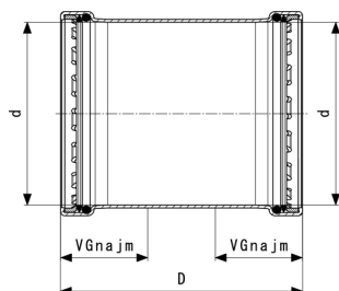
Temponox XL-Drsna spojka - nerjavno jeklo Model 1715.5XL
